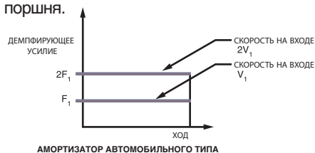
АМОРТИЗАТОР АВТОМОБИЛЬНОГО ТИПА
