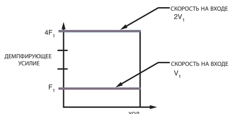
АМОРТИЗАТОР АВТОМОБИЛЬНОГО ТИПА
